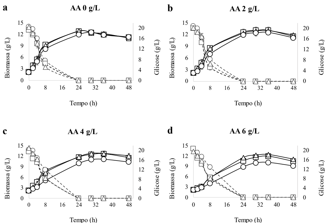
Figura 12. Perfil das linhagens de K. phaffii superexpressando Haa1 na presença de ácido acético a 0 \text{ g.L}^{-1} , 2 \text{ g.L}^{-1} , 4 \text{ g.L}^{-1} e 6 \text{ g.L}^{-1} . A produção de biomassa (linhas sólidas) e o consumo de glicose (linhas tracejadas) das linhagens de K. phaffii X33 (círculos), X33-P RPP1b -Haa1 (quadrados) e X33-P GAP -Haa1 (triângulos) estão representadas em \text{g.L}^{-1} . A: ensaio em meio controle sem ácido acético; B: ensaio em ácido acético a 2 \text{ g.L}^{-1} ; C: ensaio em ácido acético a 4 \text{ g.L}^{-1} ; D: ensaio em ácido acético a 6 \text{ g.L}^{-1} . Os valores representam a média de duas replicatas com o desvio padrão.
