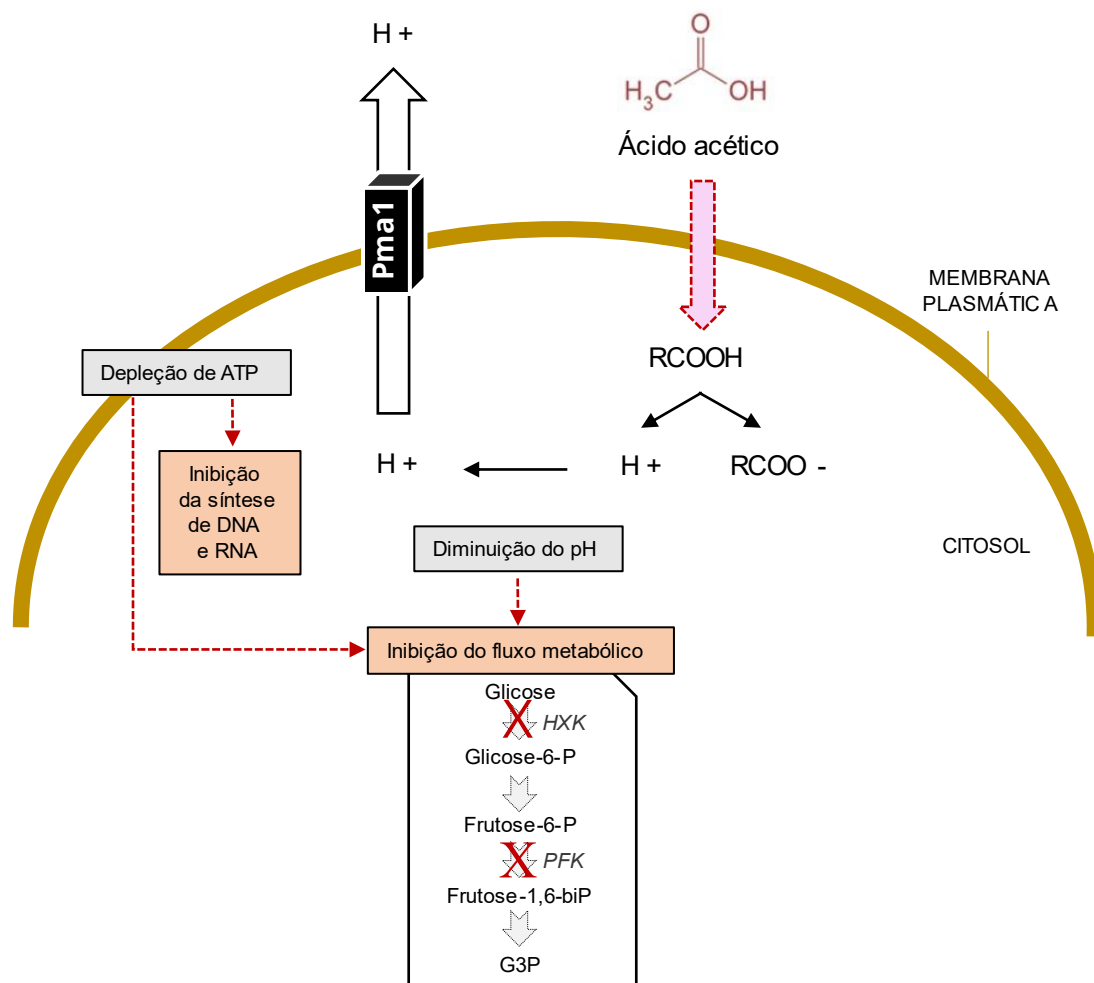
Figura 7. Efeitos inibitórios do acúmulo de ácidos orgânicos na célula. Os ácidos orgânicos (aqui representados pela fórmula “ RCOOH ”) permeiam facilmente pela membrana celular e rapidamente se dissociam no citosol devido à diferença de pH. O acúmulo de prótons é compensado pela célula pela atividade da bomba de prótons Pma1 ATPase, causando a depleção de ATP celular e a consequente diminuição de atividades essenciais, como a divisão celular e a síntese proteica, e atividade enzimática de hexoquinase (HXK) e fosfofrutoquinase (PFK). Fonte: autor.
